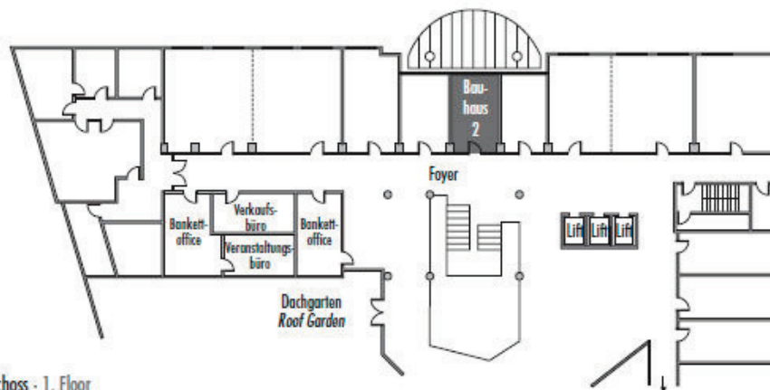
1. Obergeschoss - 1. Floor
